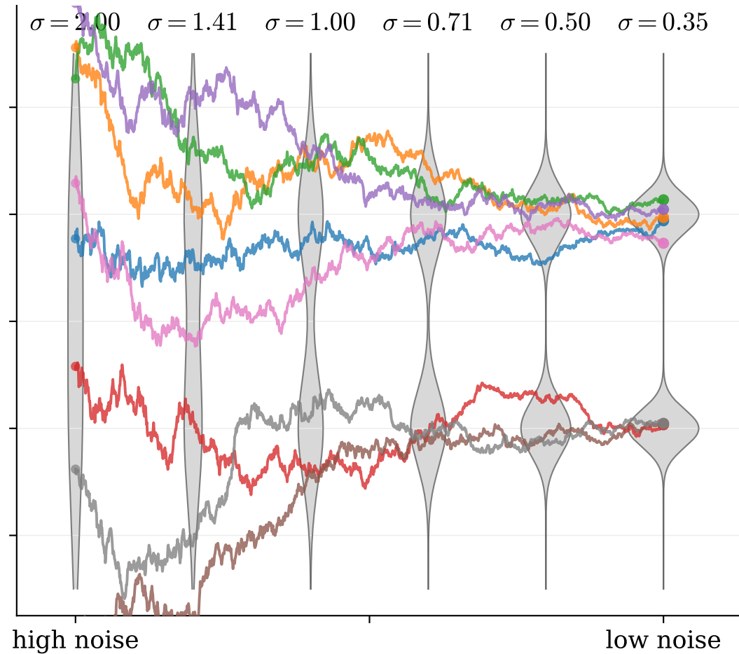
SDE Interpolation
